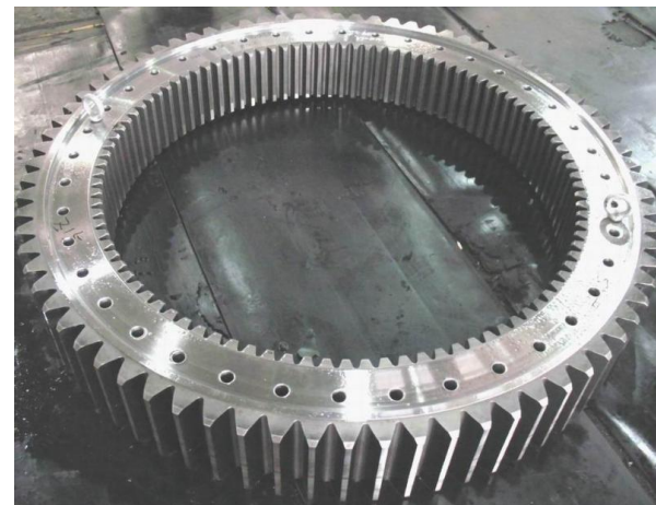
齿圈
