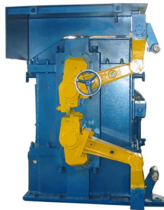
3# 飞剪
