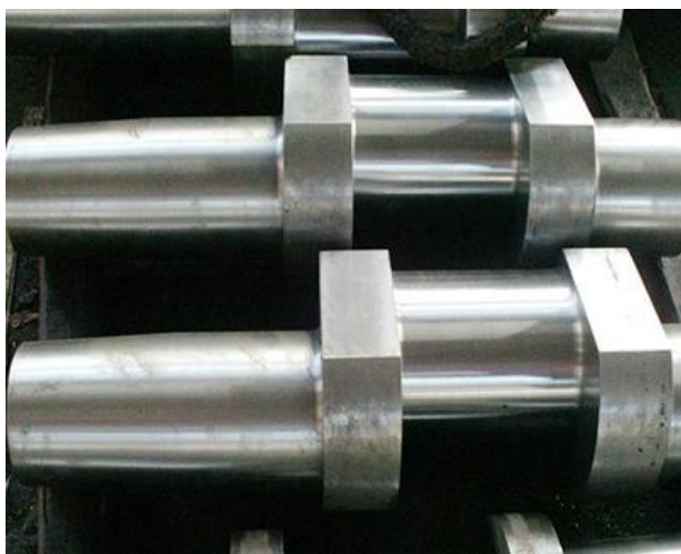
人字齿轴
